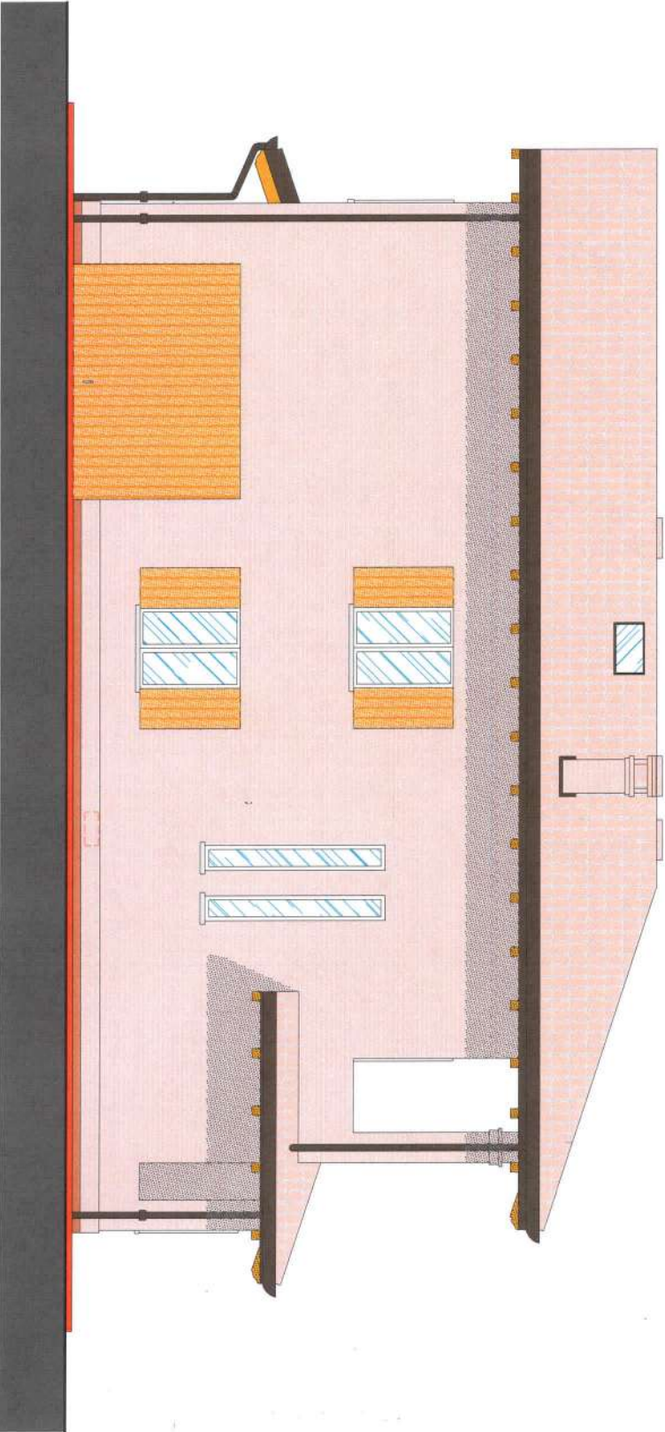
Prospetto Ovest
